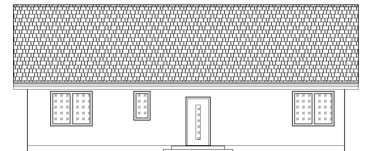
ELEWACJA PÓŁNOCNO - WSCHODNIA (FRONTOWA)
